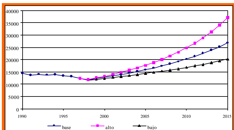
Figura 5.2. Emisiones totales de GEI por escenario de ingreso (gigagramos de CO 2 equivalente, Gg)
