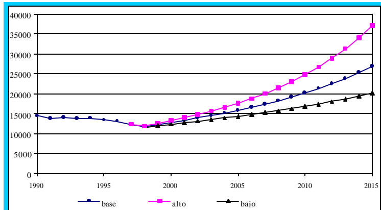
Figura 5.1.1. Emisiones totales de GEI por escenario de ingreso (gigagramos de CO 2 equivalente, Gg)
