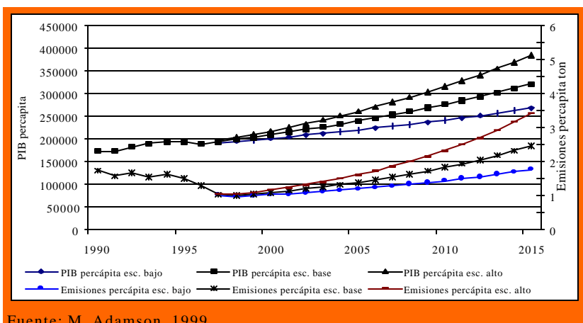
Figura 5.3 Proyecciones del PIB per cápita y emisiones per cápita de gases de efecto invernadero por escenario de ingreso 1990 – 2015 (tm y colonos de 1990)
